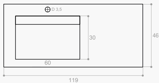
Lavabo con senos desplazados / Basins with displaced pool
